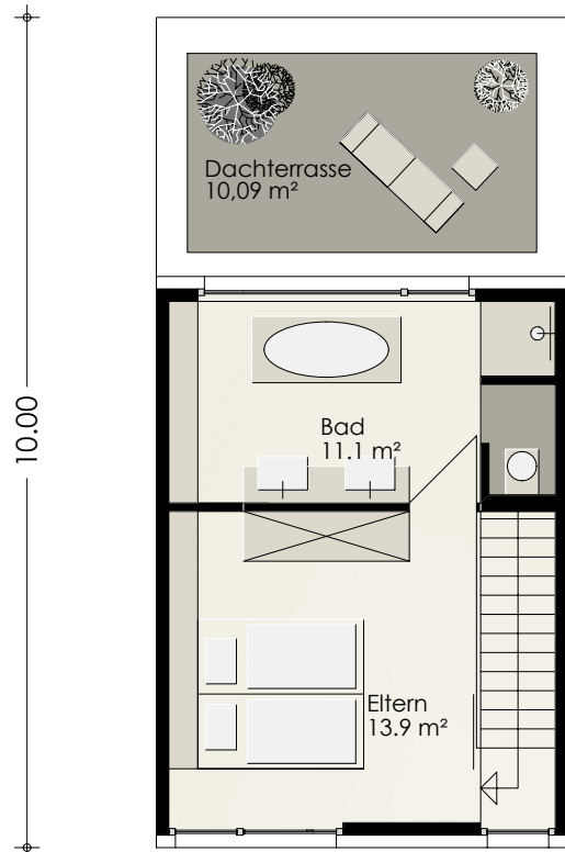
Grundriss DG, V5.2, 10 m
