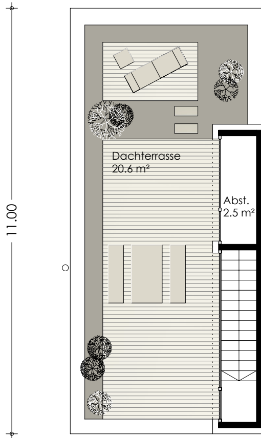
Grundriss DG, V3, 11 m
