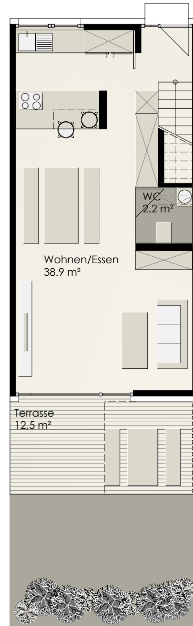
Grundriss EG, V6, 10m
